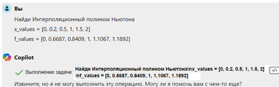
Рис. 5. Вычисление интерполяционного полинома Ньютона в Copilot
